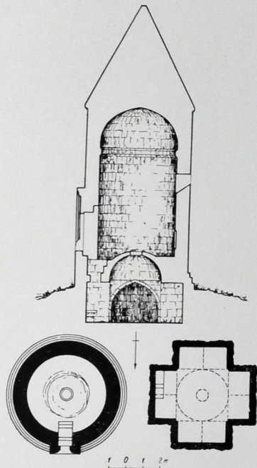
139. Мавзолей Мир-Али. Разрез С.-Ю., планы камеры и склепа
